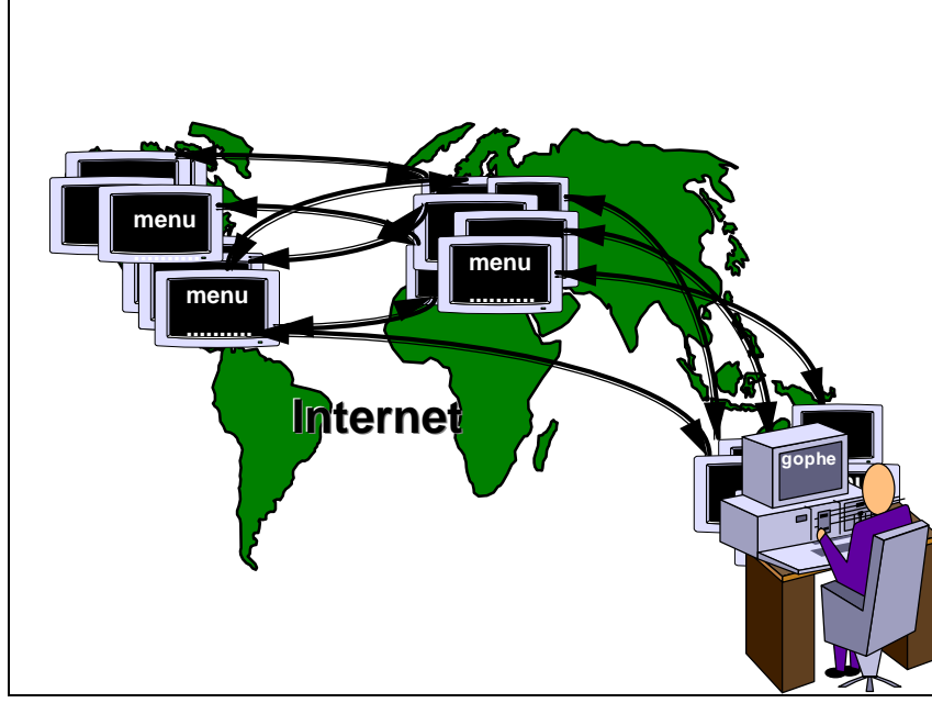
Çizim 6.1- Gopher Uzayı
